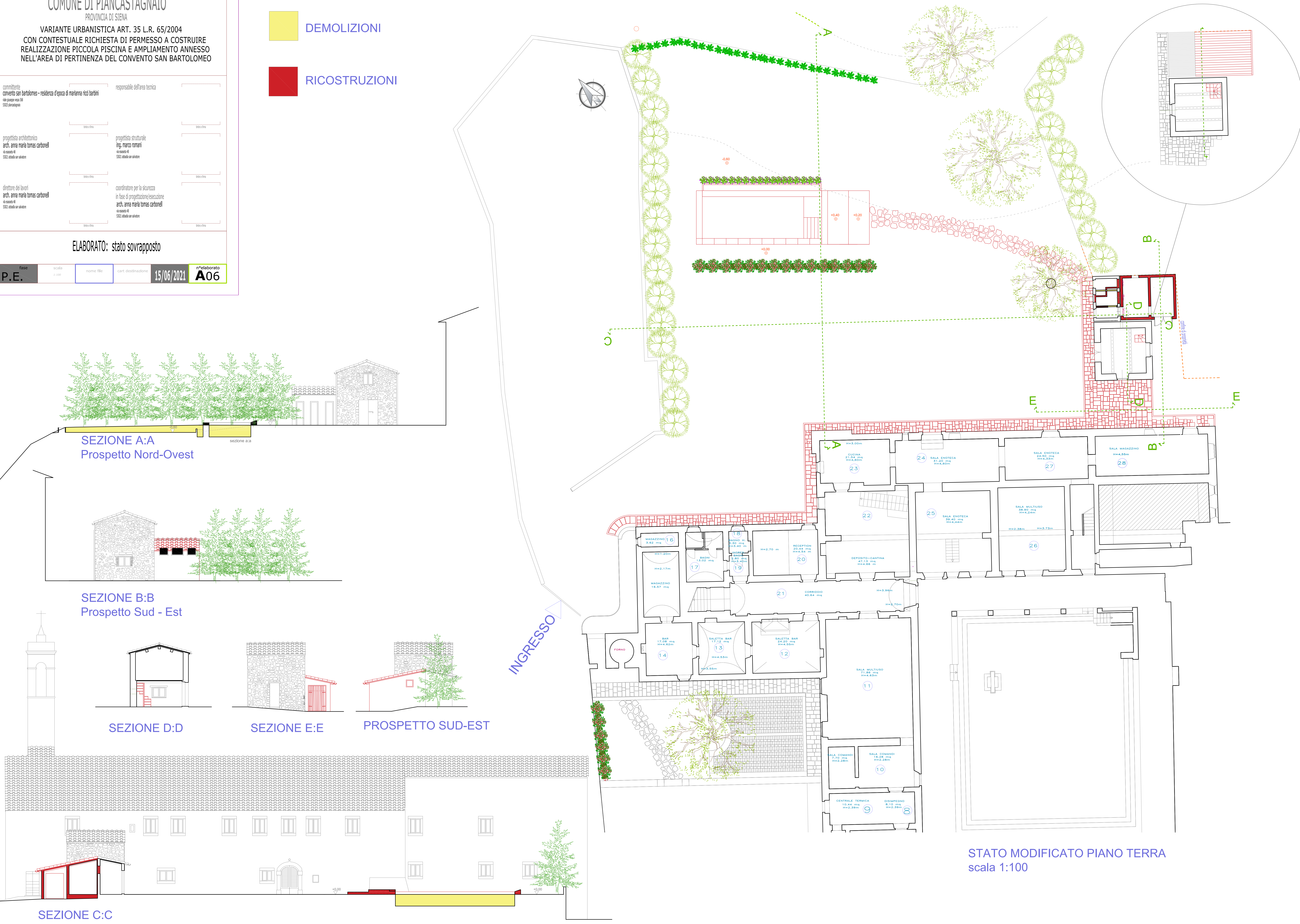
STATO MODIFICATO PIANO PRIMO scala 1:100
